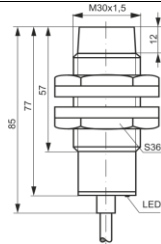
wyjście kablowe / cable output
