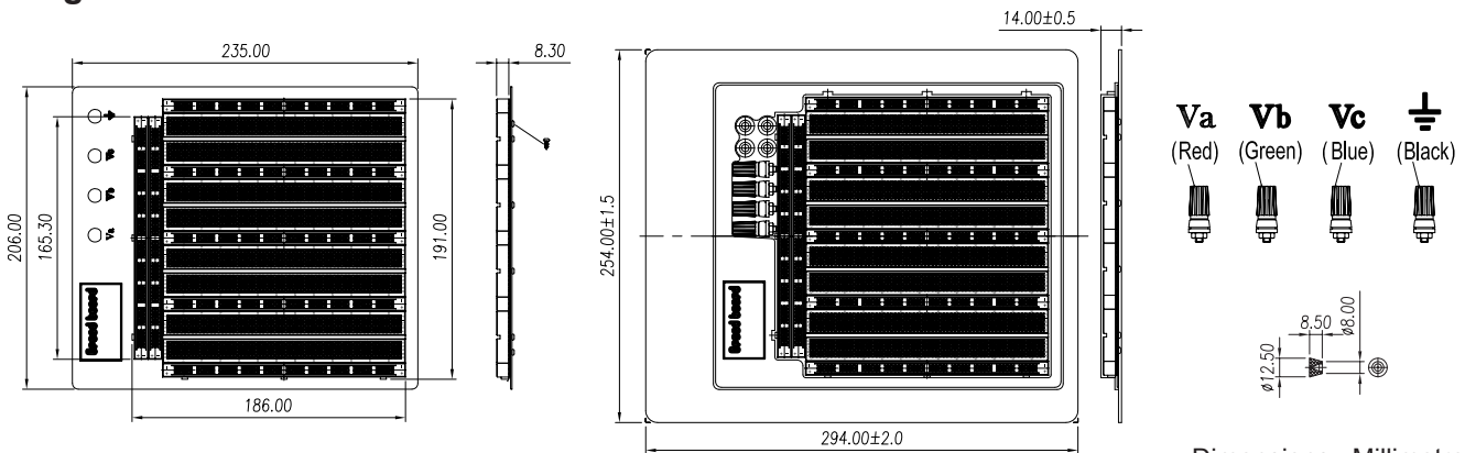
Dimensions : Millimetres
